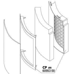
Soporte JBL CP m greenline FilterPad
