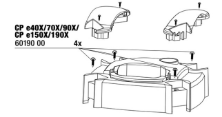
JBL CP e4/7/9/15/1900/1,2 PK vidaları
