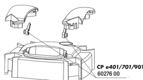
JBL CP e4/7/9/15/1901,2 Zawór odcinający, Zestaw
