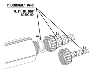
JBL PC UV-C Schlauchanschluss Set
