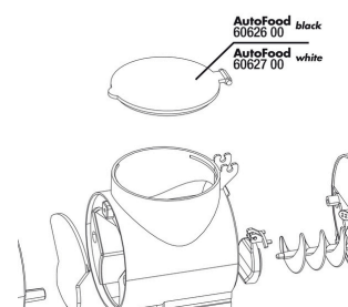
JBL AutoFood coperchio del serbatoio mangime
