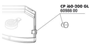
JBL CP i60-200 GL gumová podložka desky dna
