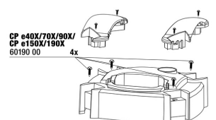
JBL CP e4/7/9/15/1900/1,2 viti testa filtro
