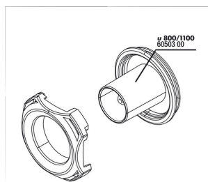
JBL PF "u" Pokrywa+ Przyłącze węża
