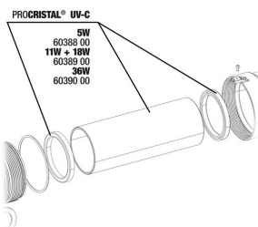
JBL PC UV-C Zestaw Ostrona szklana+ Odbłyśnik
