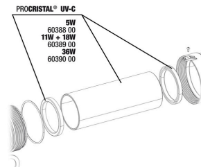
JBL PC UV-C Kit invólucro de vidro+refletor
