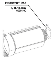
JBL PC UV-C Vedações ligação de mangueira
