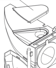
JBL CP m greenline крышка отверстия д/ выпуска воды
