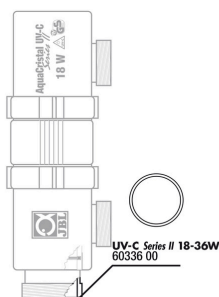
JBL AC UV-C 18/36 Вт уплотн. кольцо цилиндр.
