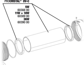
JBL PC UV-C cam manto+yansıtıcı seti
