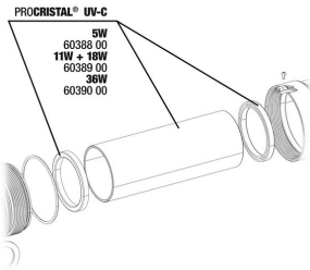
JBL PC UV-C cam manto+yansıtıcı seti
