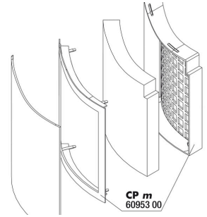
JBL CP m greenline FilterPad askı aparatı
