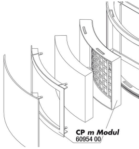
JBL CP m greenline FilterPad askı aparatı modülü
