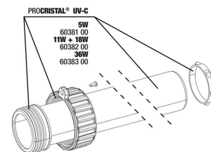
JBL PC UV-C Zestaw Bańka ze szkła kwarcowego
